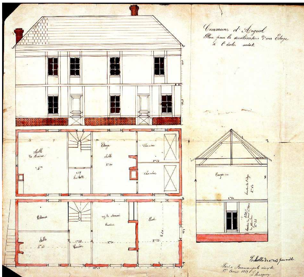
Plan de construction de l'école communale mixte, 1889 4
